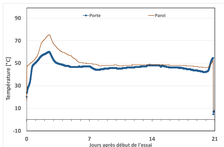
Fig. 20. Evolution de la température dans le système de méthanisation Kompoterm à Sugiez (FR) lors de l'essai de méthanisation des tubercules de souchet comestible.
